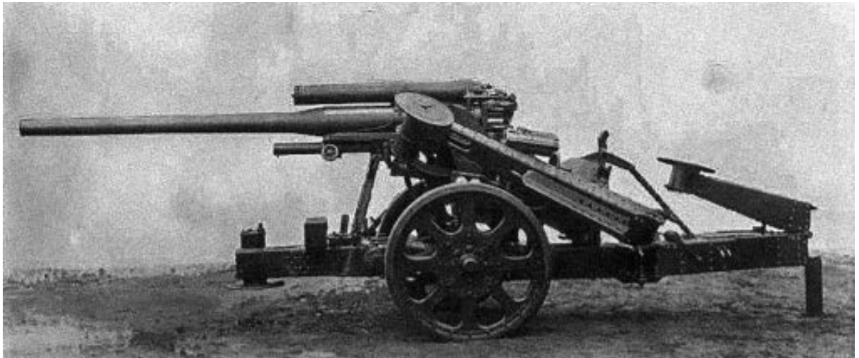
Het luchtdoelkanon van 8 cm in rijstand van de Rotterdamse firma H.I.H. Een exemplaar werd in 1929 ook beproefd, maar dat leidde door geldgebrek evenmin tot een seriebestelling.
